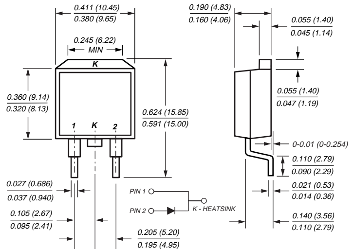
TO-263AB (DTV56B)
