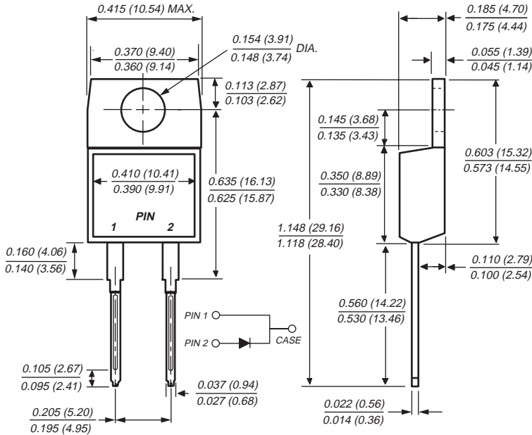
TO-220AC (DTV56)
