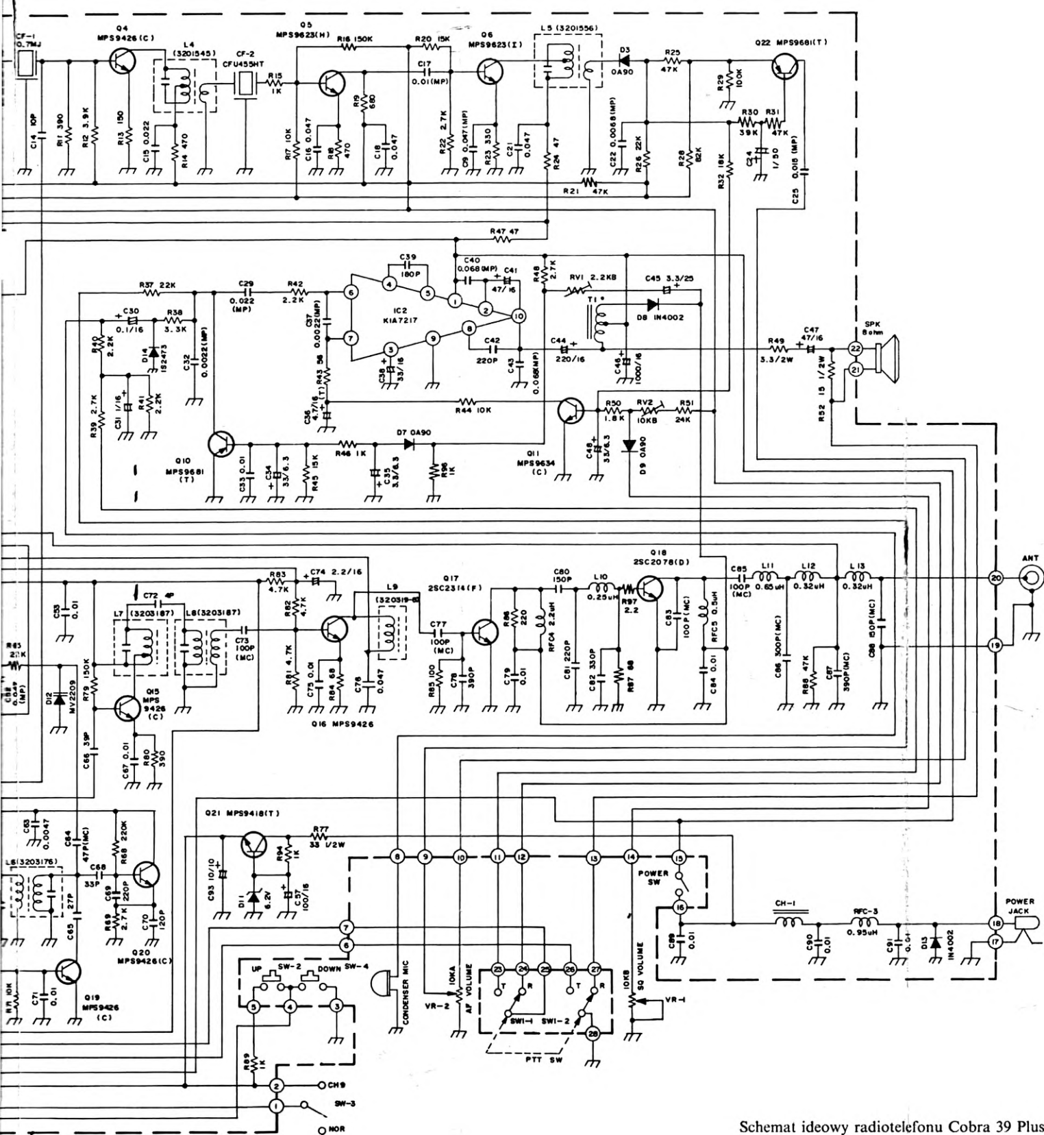
Schemat ideowy radiotelefonu Cobra 39 Plus
