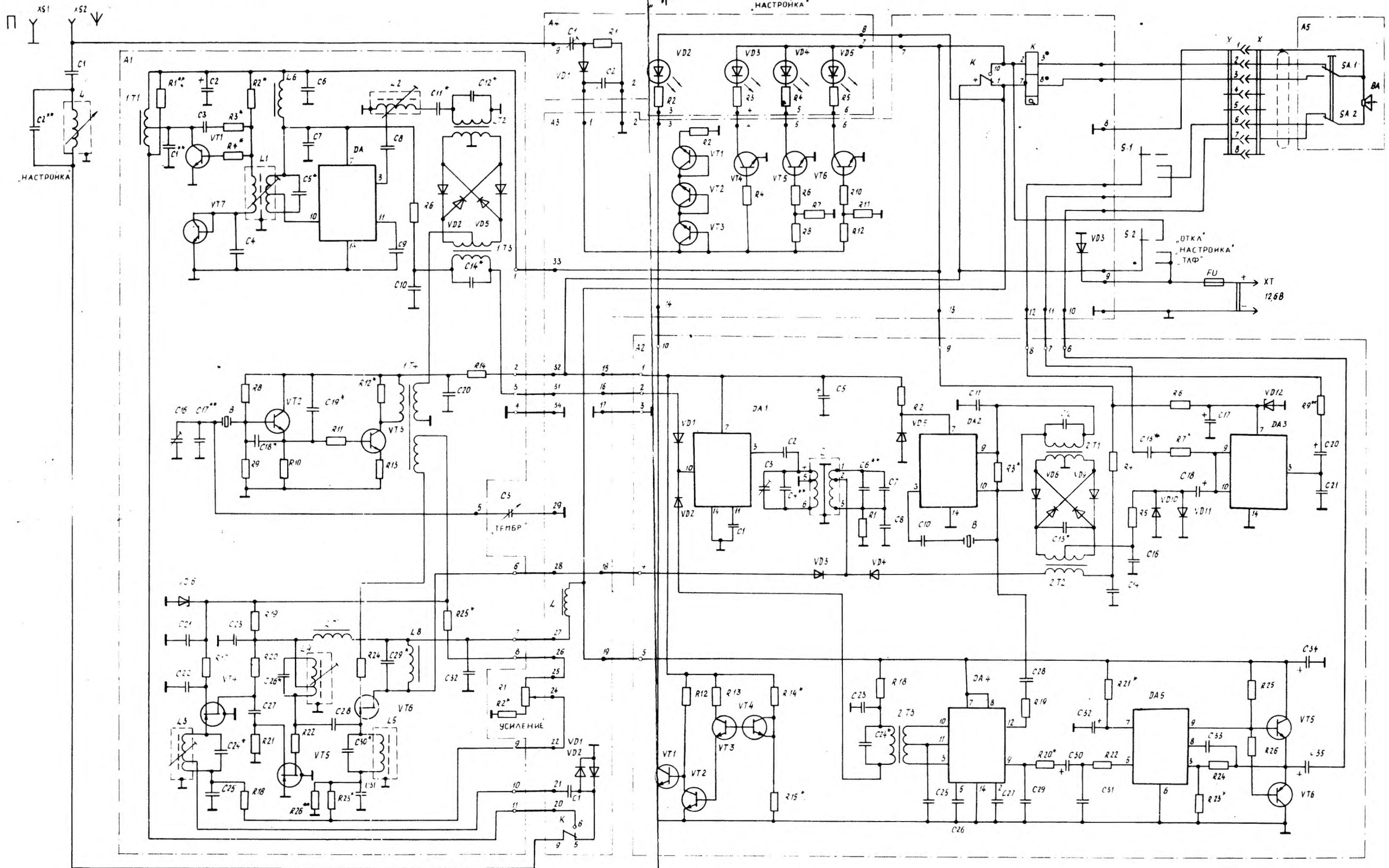
СХЕМА ЭЛЕКТРИЧЕСКАЯ ПРИНЦИПИАЛЬНАЯ ПРИЕМОПЕРЕДАТЧИКА "КАРАТ-2"
