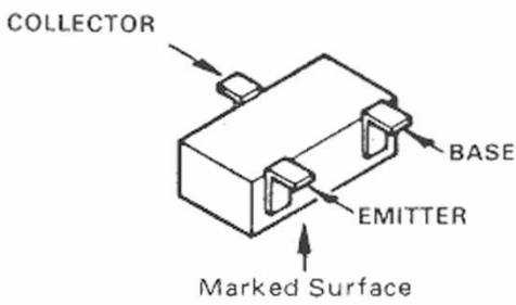
2SA1162GR(SG) (Q605, 606, 607) 2SC2712GR(LG) (Q602, 603, 608)
