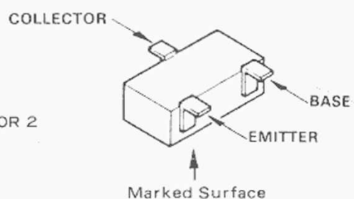
2SA1162GR(SG)(Q1004,1009) DTC144EK(26)(Q1007) 2SC2712GR(LG)(Q1008) DTC124TK(05)(Q1010)
