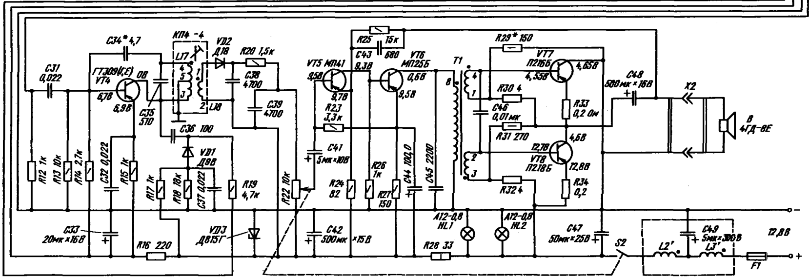
Принципиальная электрическая схема радиоприемника А-370 (А-370М, А-370М1)
