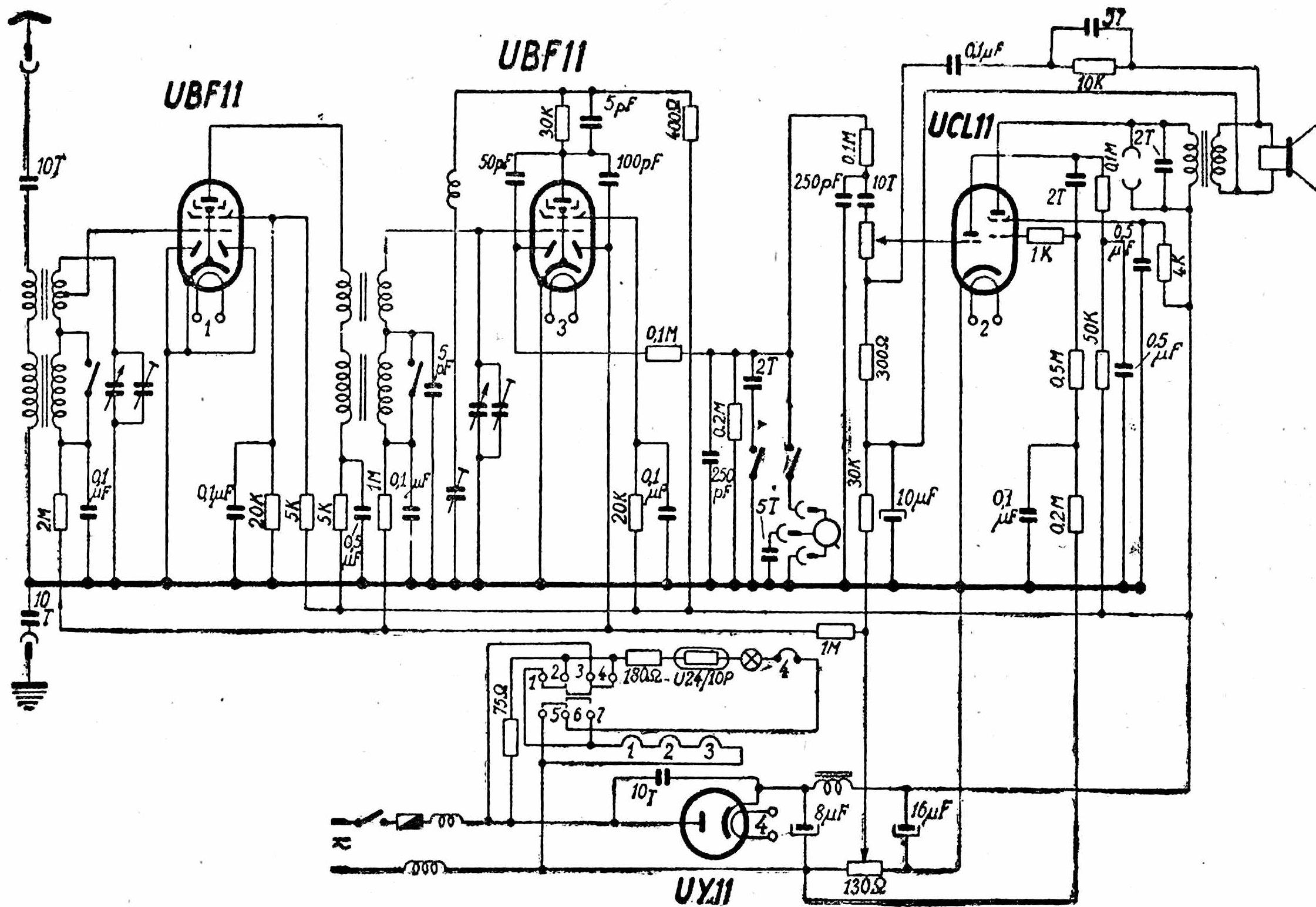
Schemat odbiornika uniwersalnego AEG 29 GW.
