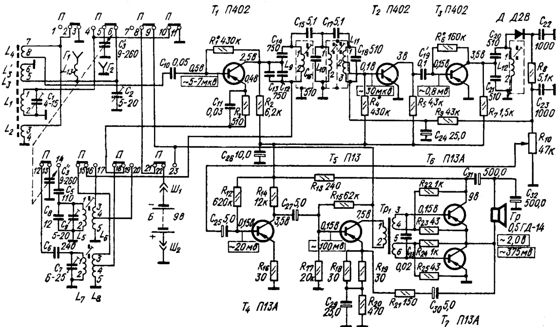
Принципиальная электрическая схема радиоприемников «Атмосфера» (переключатель диапазонов в СВ)
