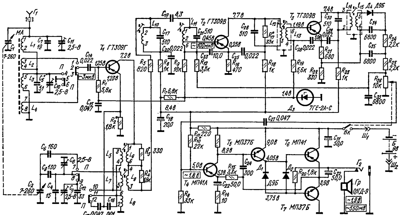
Принципиальная электрическая схема радиоприемников (переключатель диапазонов в положении ДВ).
