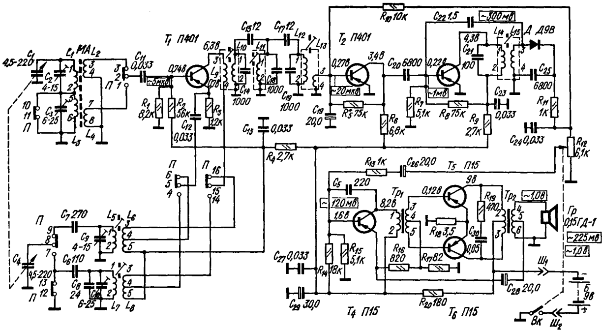
Принципиальная электрическая схема радиоприемника «Гауя» (переключатель диапазонов в положении СВ).
