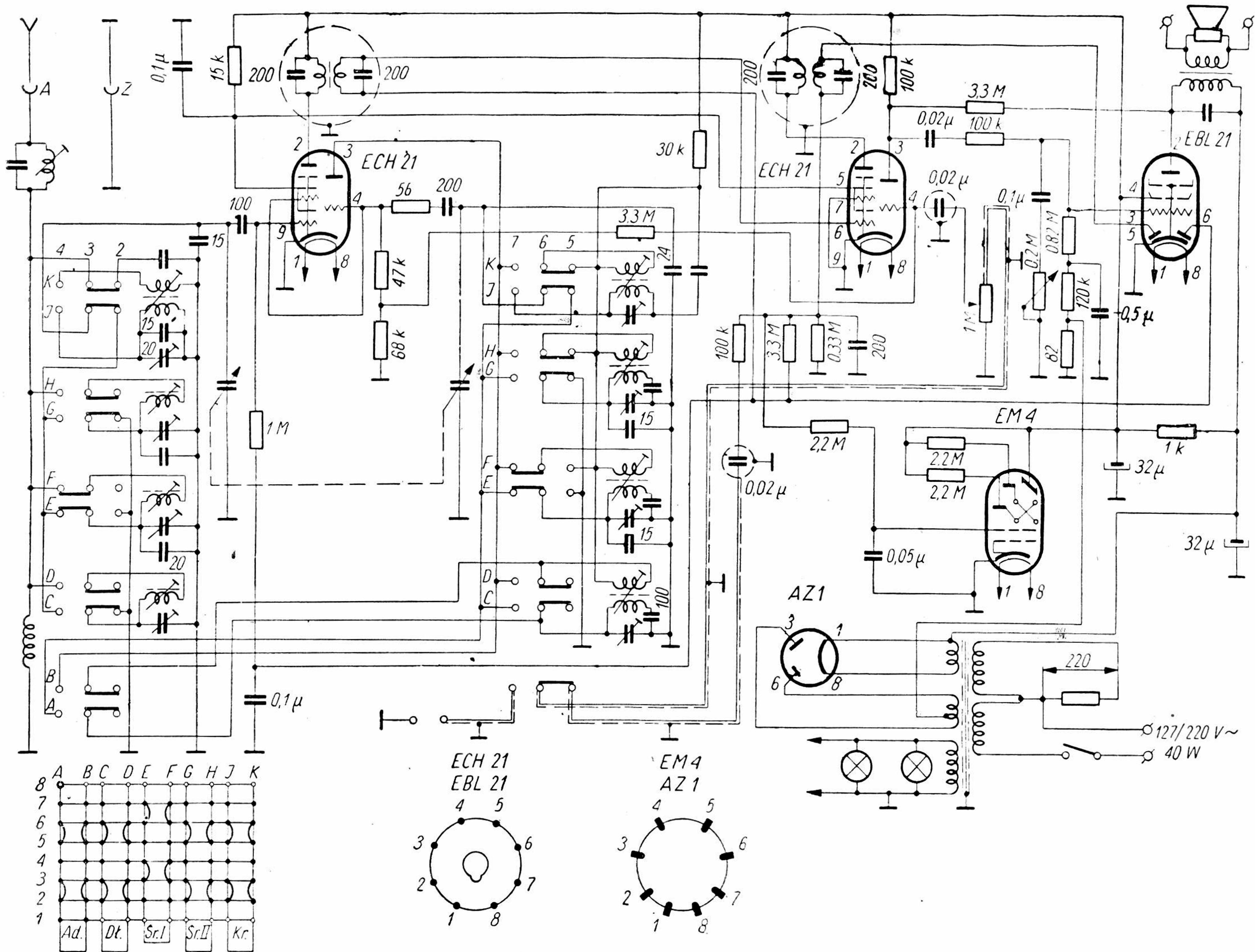
Schemat ideowy odbiornika „Kaprys“
