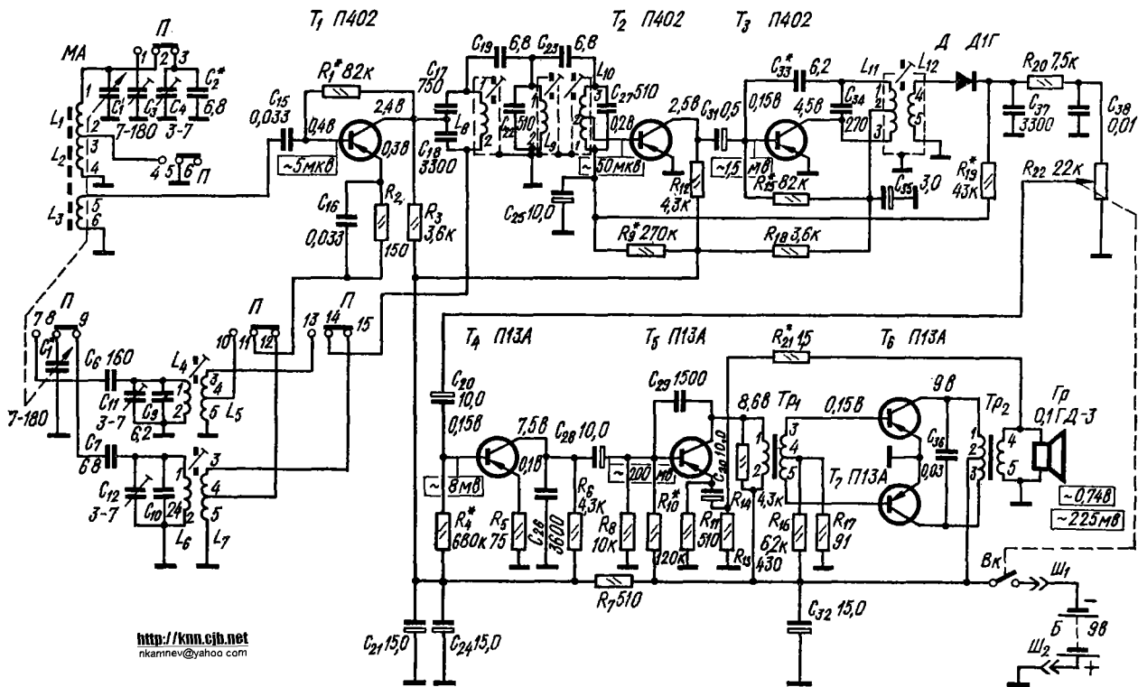
Принципиальная электрическая схема радиоприемников «Ласточка» (Б) (пе рклячатель диапазонов в полож. ДВ)
