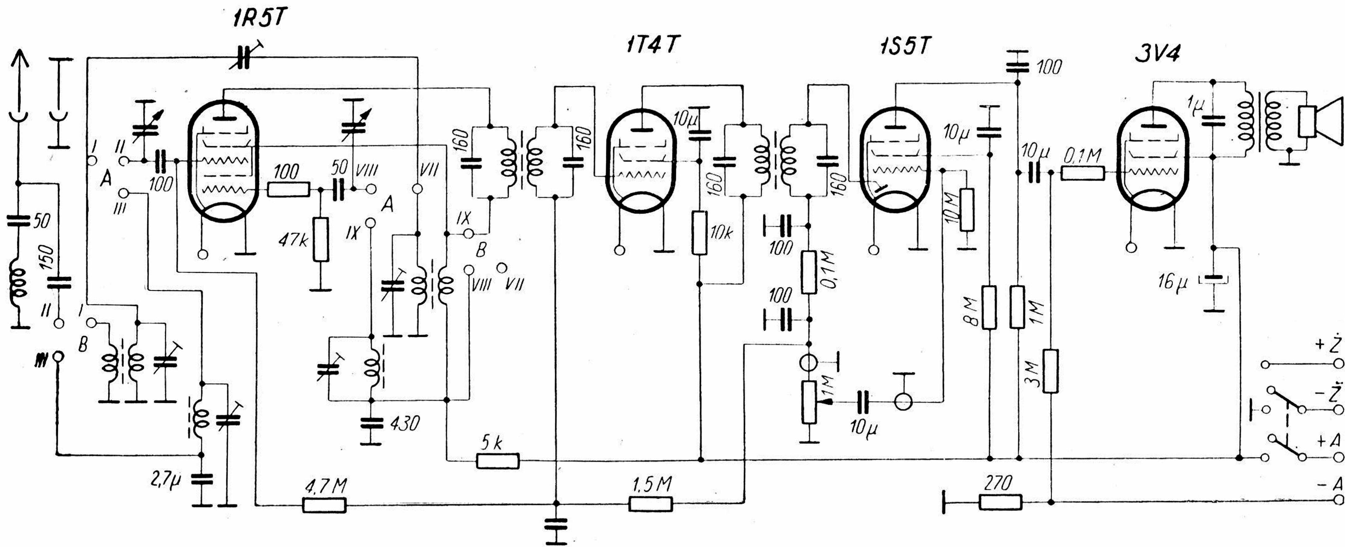
Schemat ideowy odbiornika Orion B646
