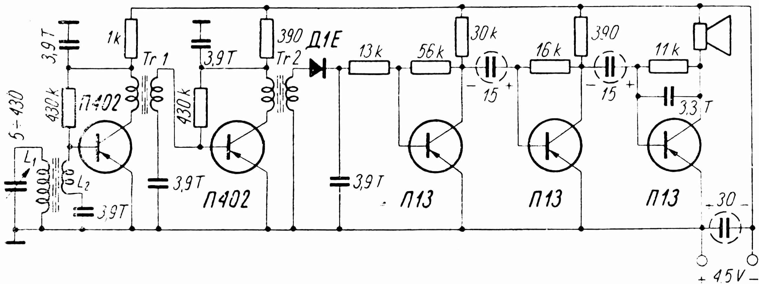
Schemat odbiornika „Sputnik“
