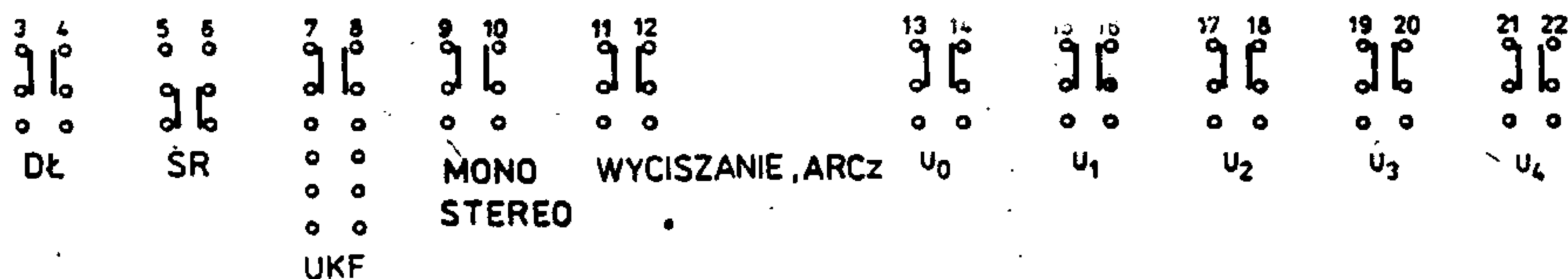
Schemat ideowy tunera stereofonicznego Hi-Fi typu AS-618
